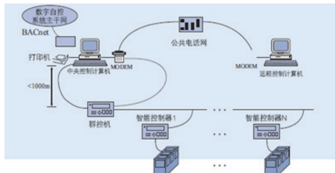
网络控制系统示意图
