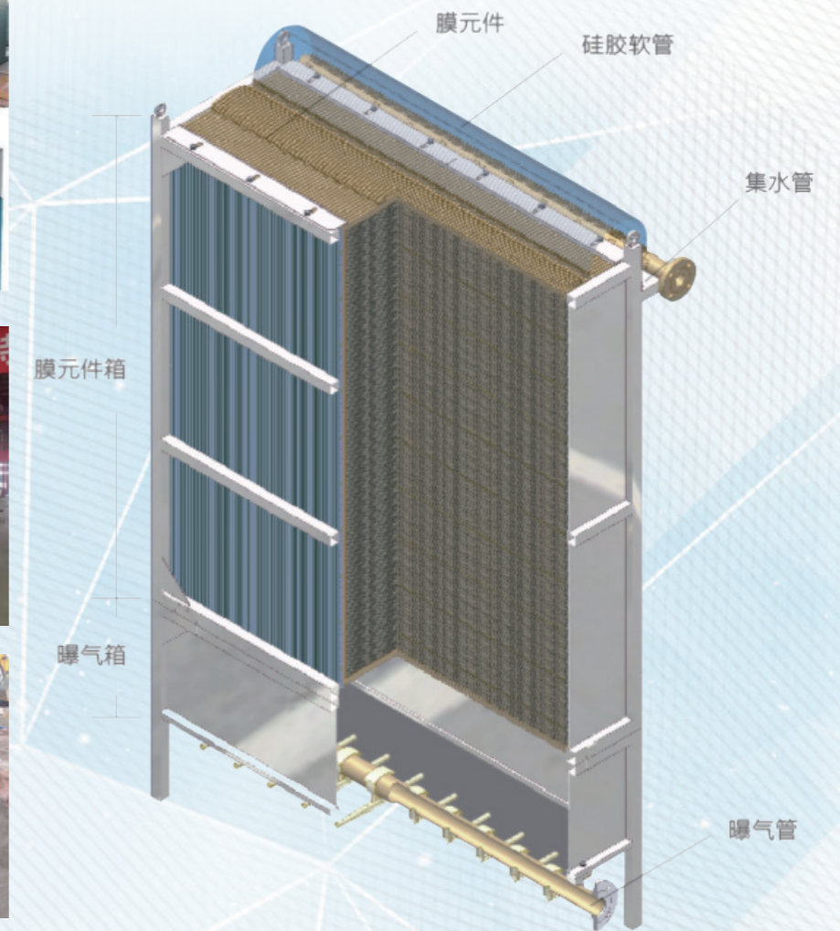
膜组件结构图
